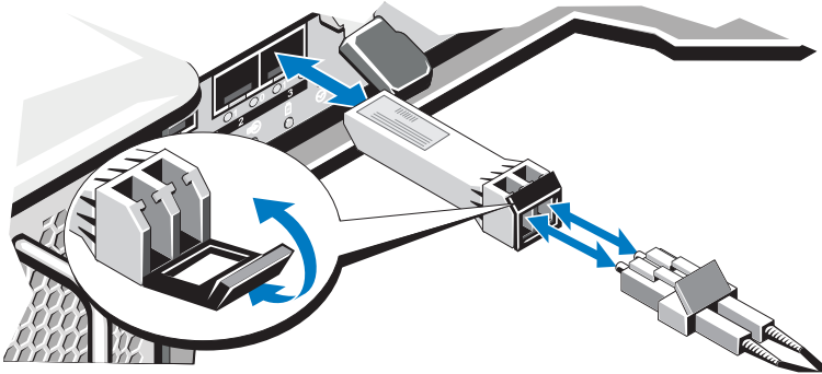
图 20-1. 移除 SFP 模块
